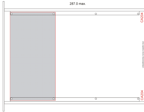
Quereinbau von Leiterplatten mit Zubehör CA204 Kundenspezifische Bearbeitung von CA204 ist möglich.
