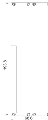
Rückwand CA214 1 Stück
