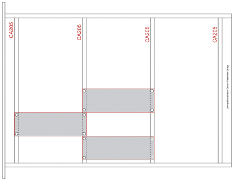
Längseinbau von Leiterplatten mittels Zubehör CA205. Kundenspezifische Bearbeitung von CA205 ist möglich.
