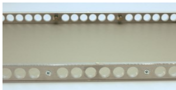
CAMAC-Zusammenbau-b2
