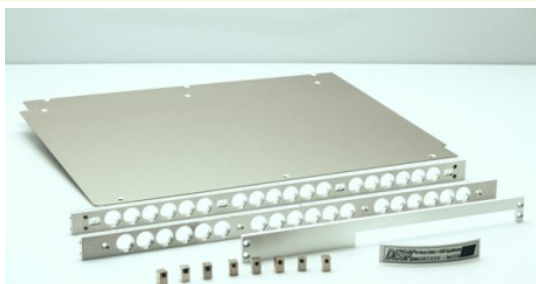
CAMAC1-25-Einzelteile
