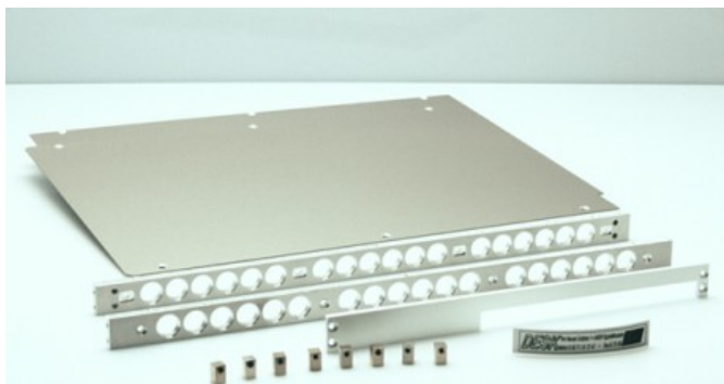
CAMAC1-25-Einzelteile Nicht dargestellt sind die Schrauben!
