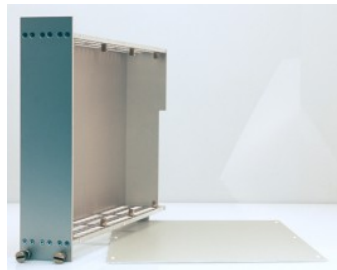
CAMAC3-25-Komplett
