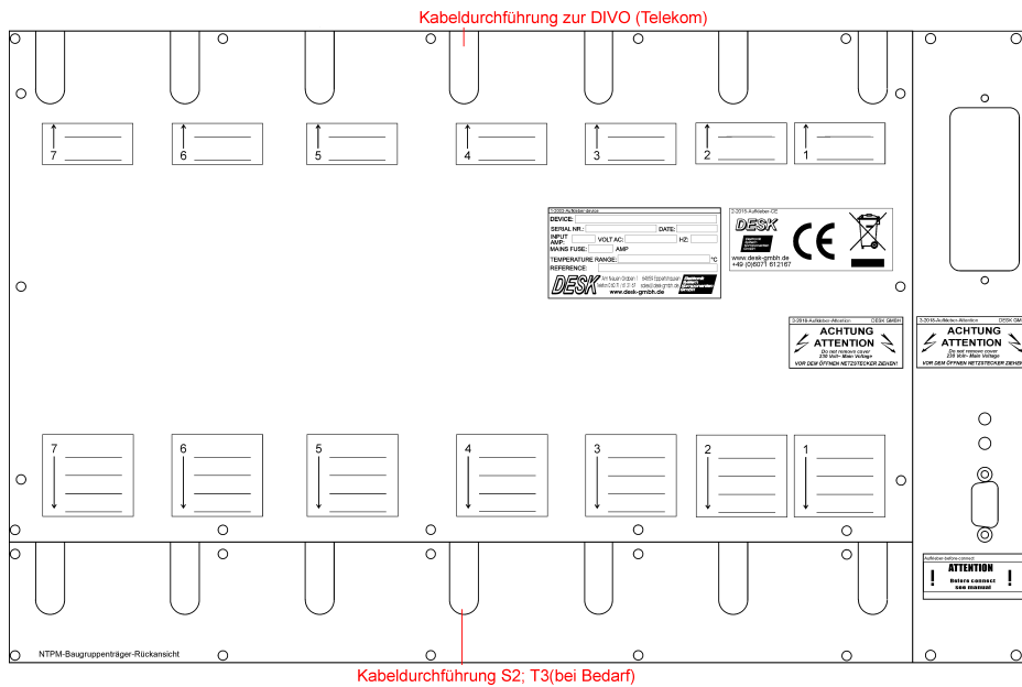
Rückansicht der Netzteile
