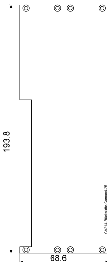
CAMAC 4/25 Rückplatte Art. Nr. CA214 Rückplatte für CAMAC 4/25 Cassette Material: AlMg3 Oberfläche: Gebürstet oder chromatiert Natur Lieferzeit: ab Lager
