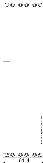
CAMAC 3/25 Rückplatte Art. Nr. CA215 Rückplatte für CAMAC 3/25 Cassette Material: AlMg3 Eloxalqualität Oberfläche: Gebürstet oder chromatiert Natur Lieferzeit: ab Lager
