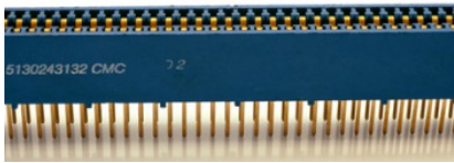
Federleiste CAMAC3
