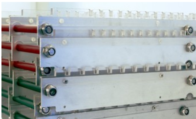
Frontplattenständer
