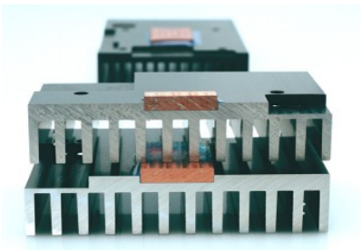
Kühlkörper-mit-Kupferinlay
