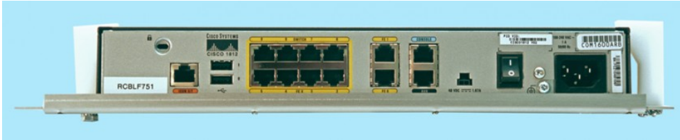
Einbaubeispiel für Geräte der Cisco Series 18xx. Diese Geräteserie markiert die Maximalabmessungen der einzubauenden Geräte: B = 343 mm T = 274 mm H = 48 mm
