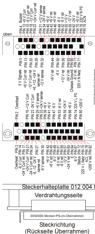
Stecker im NIM Überrahmen , Einbau und Lage der Anschlüsse
