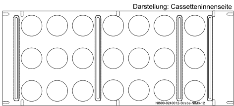
Strebe oben/unten NI600 / 024 001 2 2 Stück
