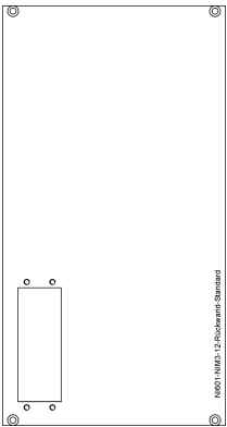
Rückwand NI601 1 Stück
