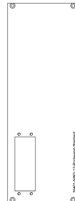
Rückwand NI401 1 Stück
