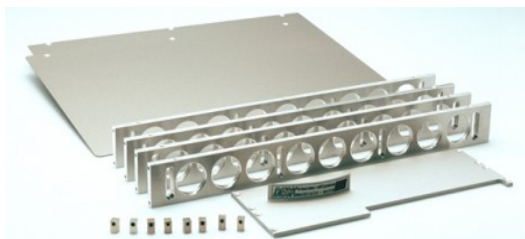
CAMAC4-25-Einzelteile
