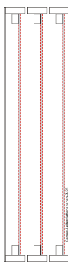
CAMAC 3/25 Einbaumöglichkeit für drei Leiterplatteebenen (Grundposition im Raster 17.2 mm).
