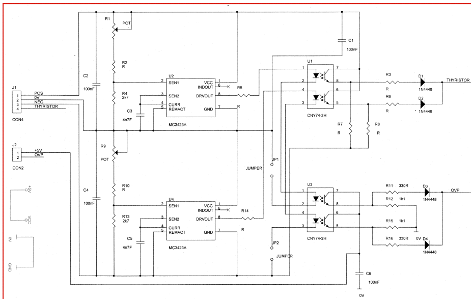
Stromlaufplan-OVP
