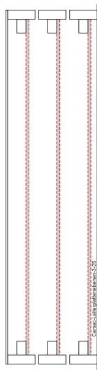
CAMAC 3/25 Einbaumöglichkeit für drei Leiterplattenebenen (Grundposition im Raster 17.2 mm).
