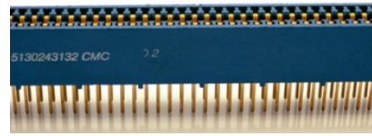
Federleiste CAMAC3
