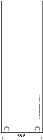
Abdeckstreifen CAMAC 4/25 Art. Nr. CA210
