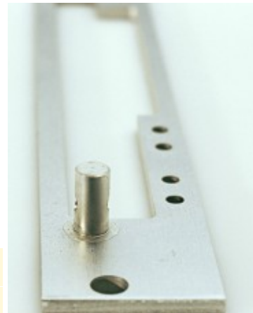
Leiterplattenbefestigung-Einpreßbolzen
