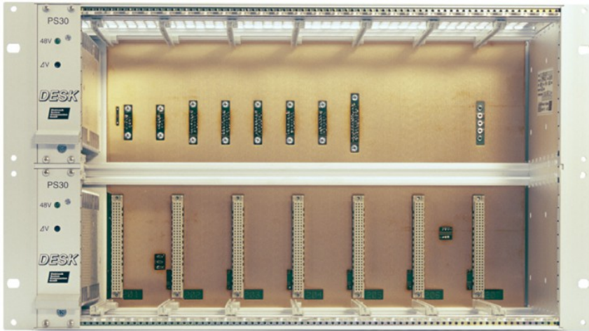
DESK_GmbH_2013-16B062-6HE-Baugruppenträger
