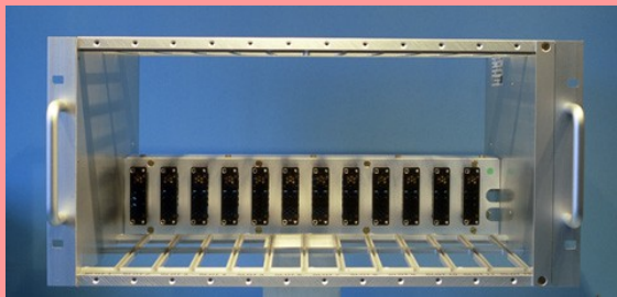
DESK_GmbH_1-B017-NIM-Überrahmen
