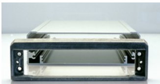
Druckgussblende + Strangpressprofil
